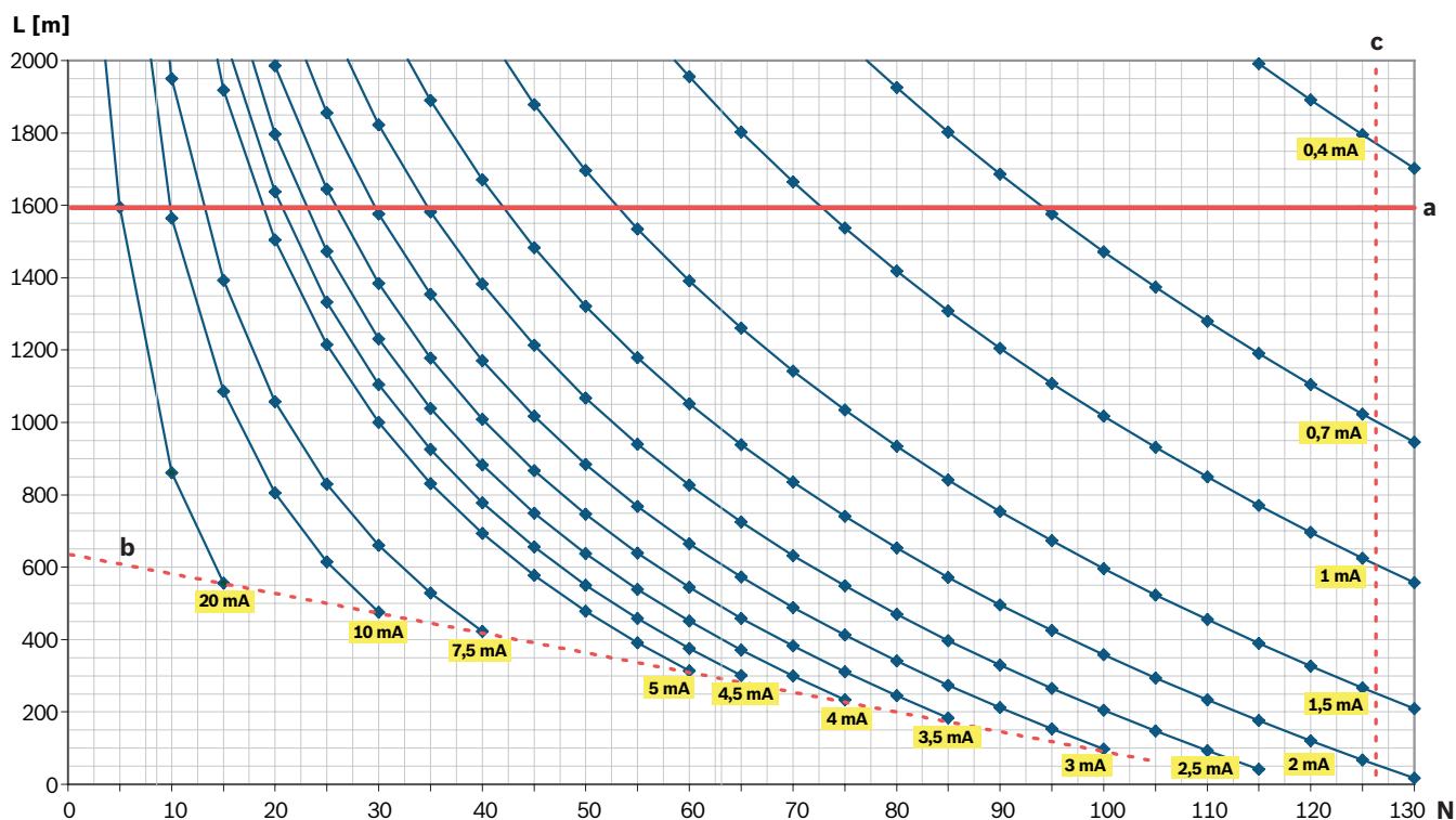
Rysunek 3.1: Schemat określania maksymalnej dozwolonej długości kabla: elementy w technologii LSN classic z modułem LSN 0300 A
