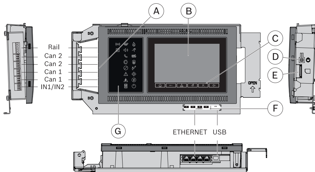
Rysunek 2.2: Przegląd kontrolerów central
