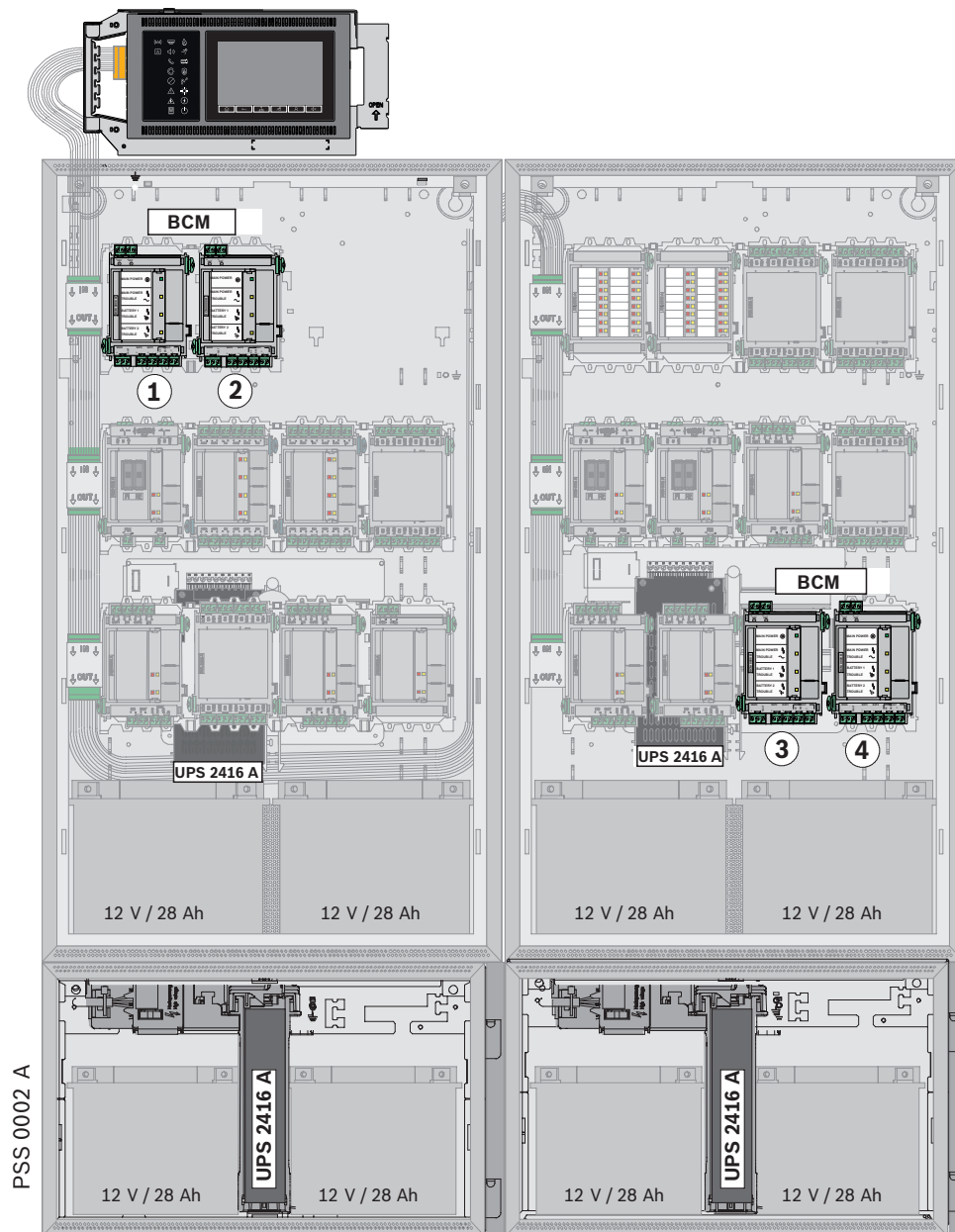
Rysunek 3.5: Konfiguracja z 1-4 modułami BCM (montaż ścienny)
