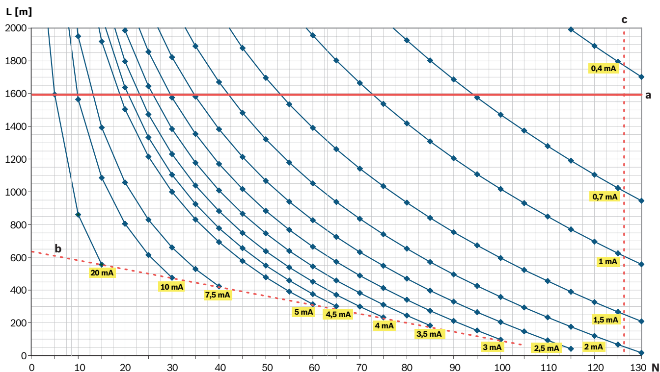
Рис. 3.1: Диаграмма для определения максимально допустимой длины кабеля: элементы LSN classic с LSN 0300 A
